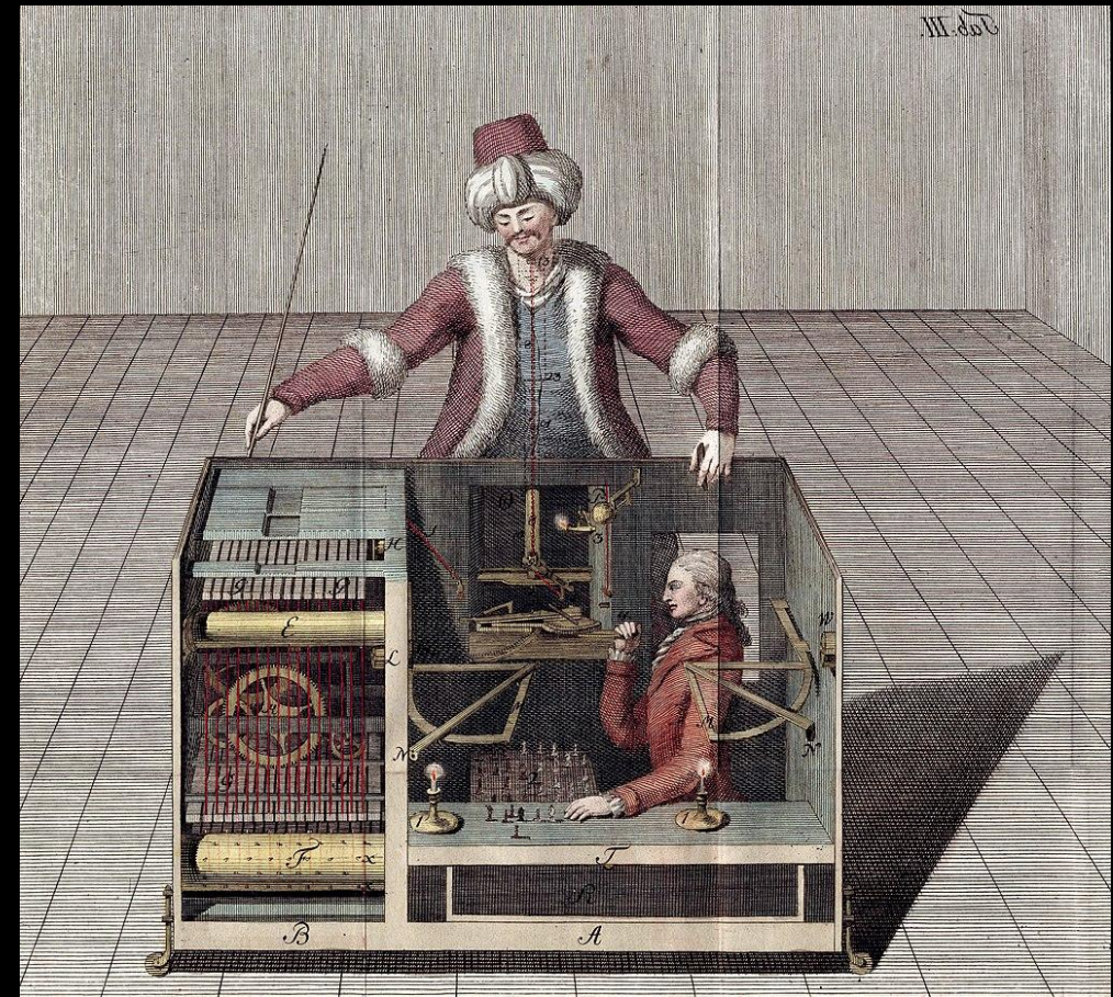
Et tværsnit af "skaktyrkeren" fra Racknitz, som dog tog fejl både med hensyn til operatørens position og automatens dimensioner.
